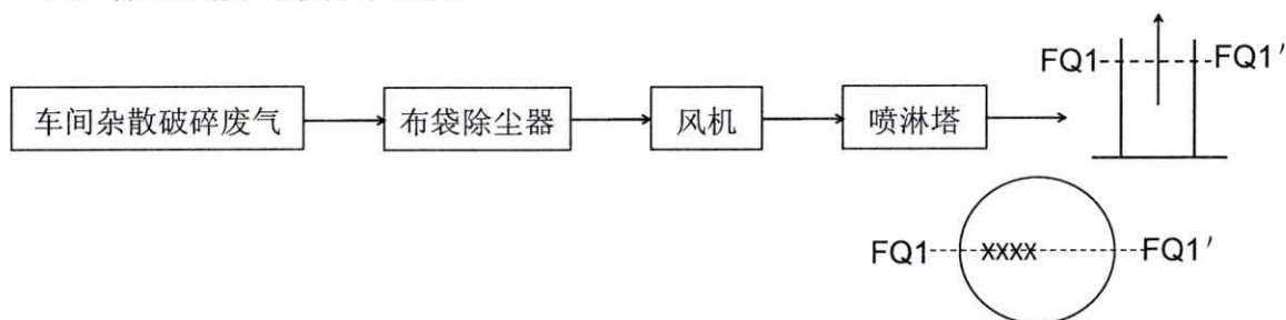
图 2 有组织废气采样点示意图
